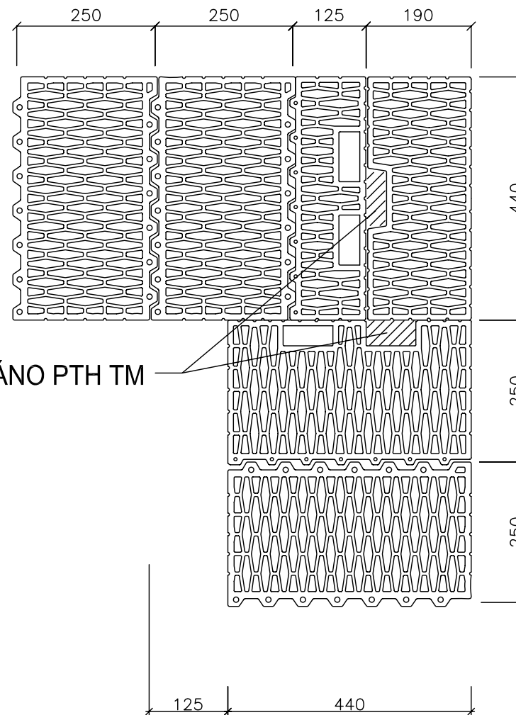
POROTHERM 44 P+D VAZBA ROHU
