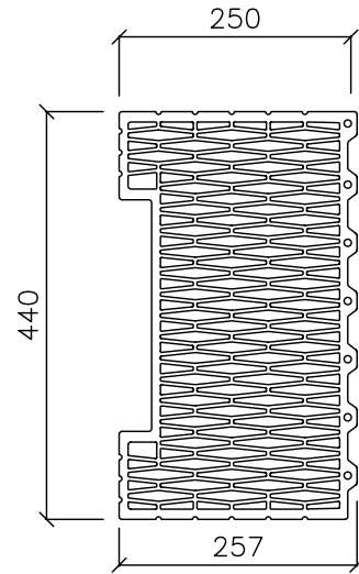
POROTHERM 44 K Si
