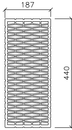
POROTHERM 44 R Si
