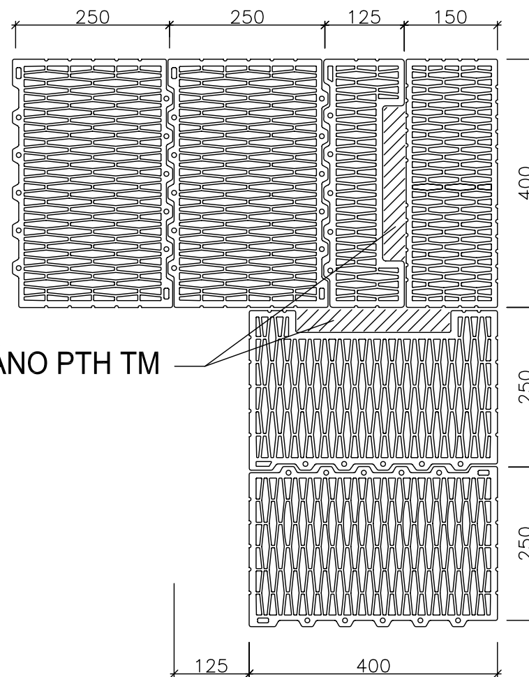
POROTHERM 40 Si VAZBA ROHU
