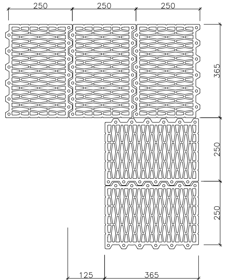
POROTHERM 36,5 P+D VAZBA ROHU
