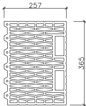
POROTHERM 36,5 K
