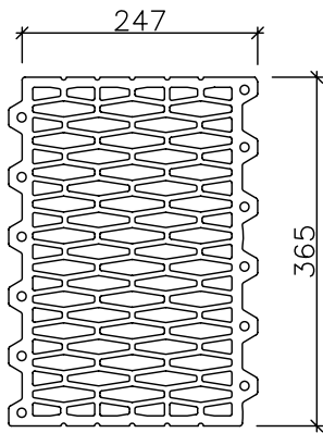
POROTHERM 36,5 P+D
