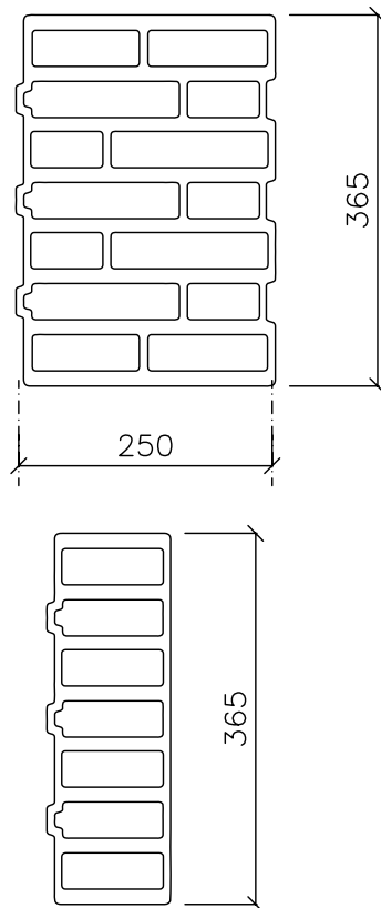
POROTHERM 36,5 Ti
