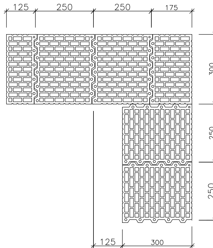
POROTHERM 30 P+D (CB) VAZBA ROHU
