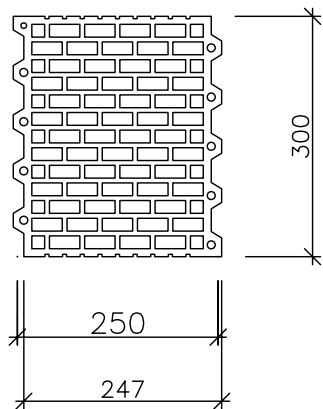
POROTHERM 30 P+D (CB)
