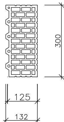
POROTHERM 30 1/2 P+D (CB)
